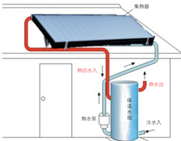
(圖二) 太陽能熱水系統
