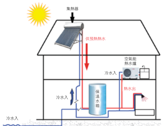
(圖三) 太陽能空氣能混合熱水系統
