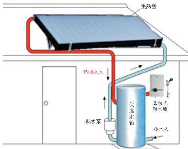
(圖四) 太陽能電能混合熱水系統
