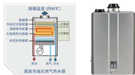
(圖三) 燃氣即熱式熱水爐
