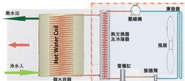
（圖四）空氣能熱水爐（熱泵）運作原理
