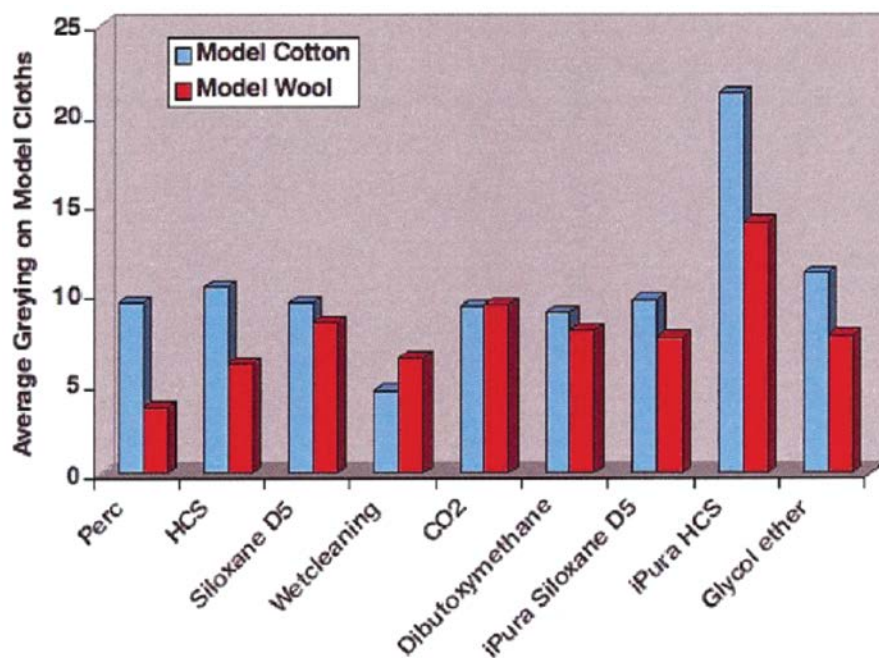
圖3：顯示經過各種溶劑及機器技術作三次清洗後，造成標準試驗樣布顏色灰暗平均值
