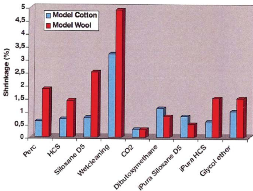
圖2：顯視標準試樣布在3次清洗後的收縮率
