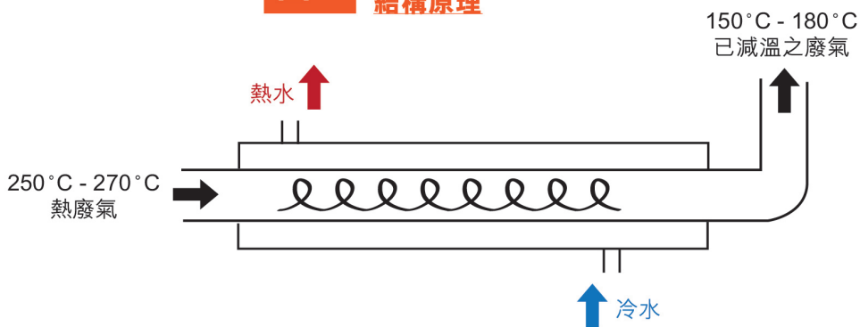
圖二 管道式密封儲水箱的結構原理
