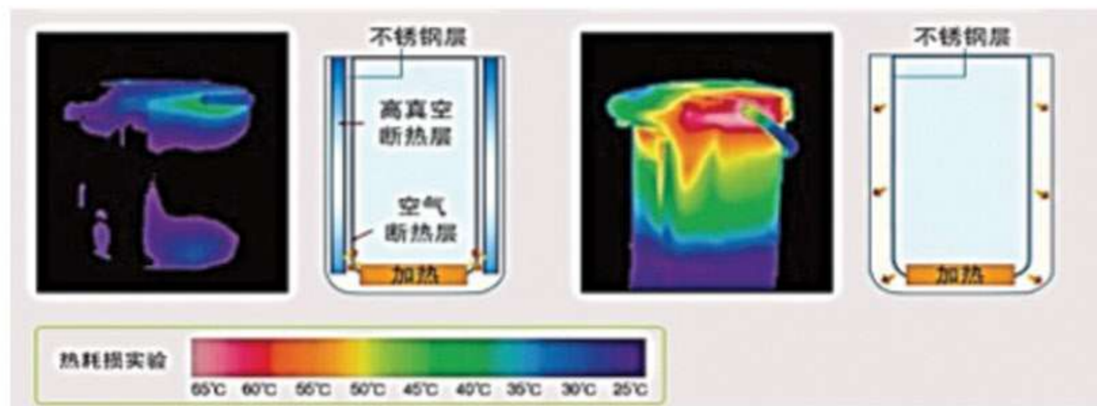
圖四：真空斷熱及一般保溫外殼溫度比較圖
