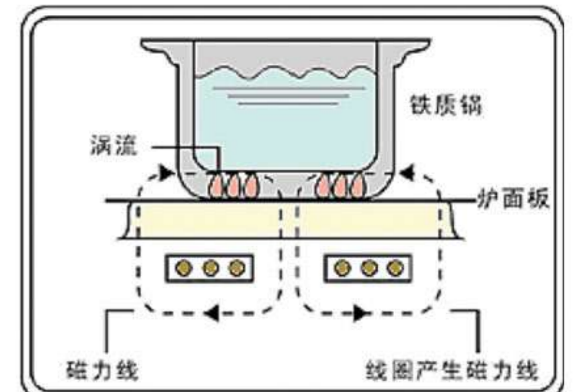
圖二：電磁感應加熱原理
