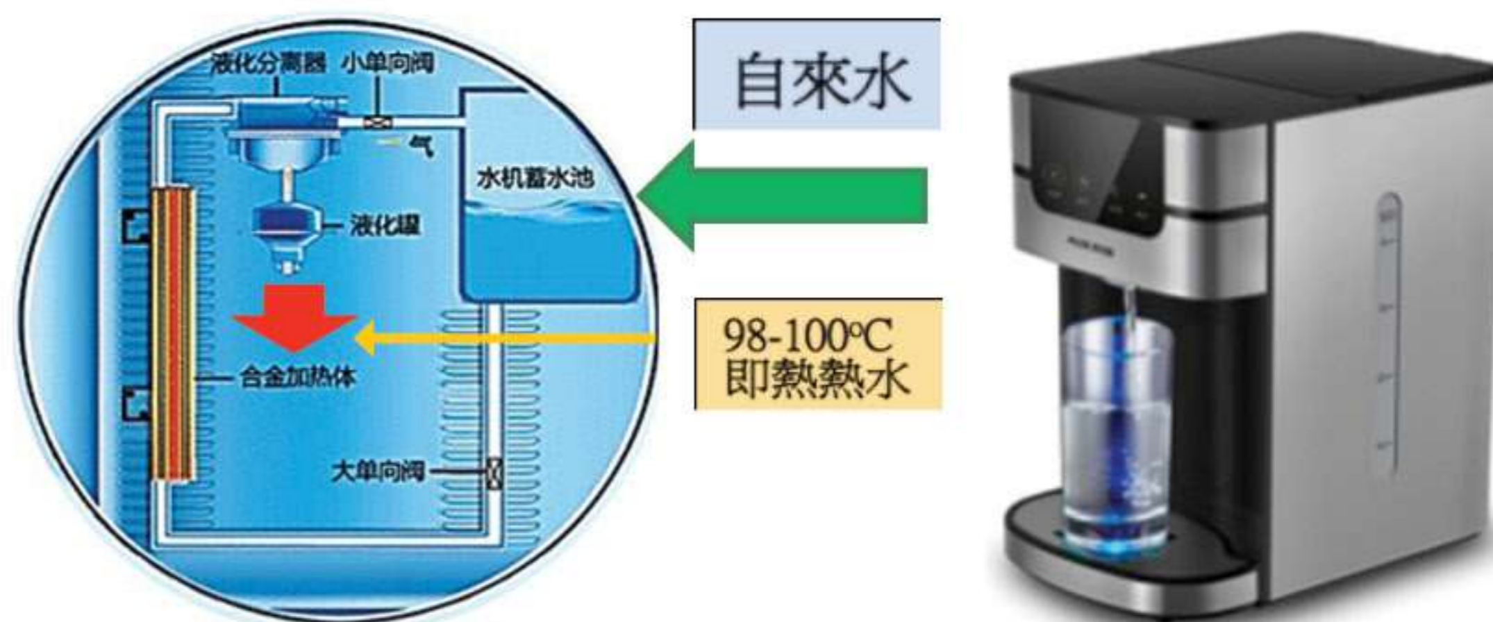
圖五：即熱式電熱水瓶原理
